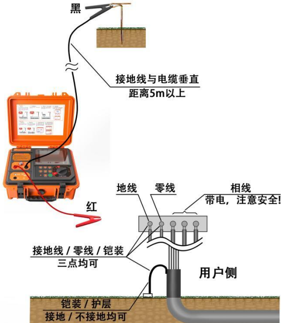
图 5- 20 运行电缆零线 / 地线 / 护层注入法
