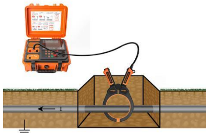
图 5-14 卡钳耦合合法接线图
