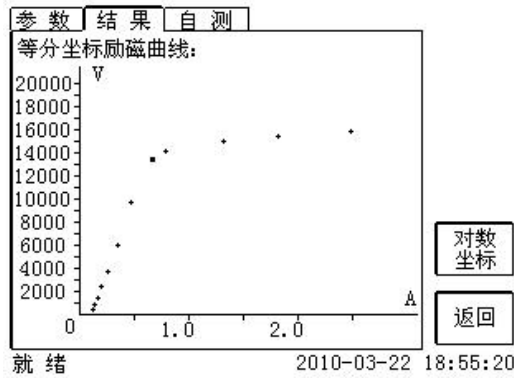
图 2.19 励磁曲线界面
