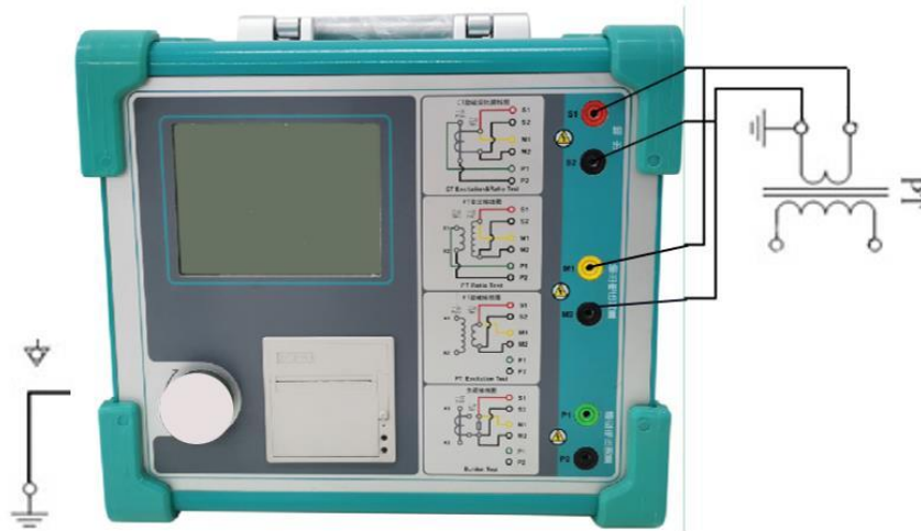
图 2.7 PT 直阻、励磁试验接线方式
