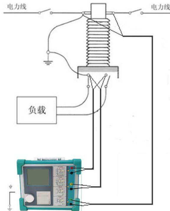
图 C.1 典型接线方式
