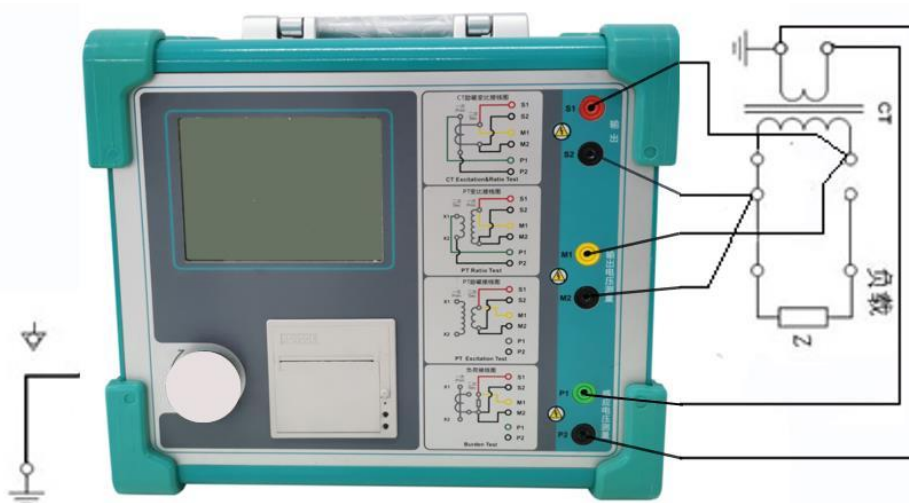
图 2.1 CT 直阻、励磁、变比试验接线方式
