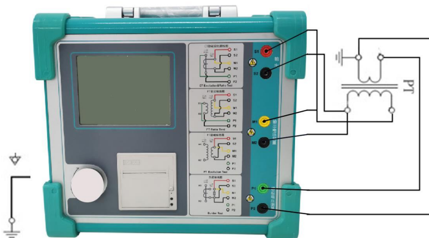
图 2.8 PT 变比、极性试验接线方式
