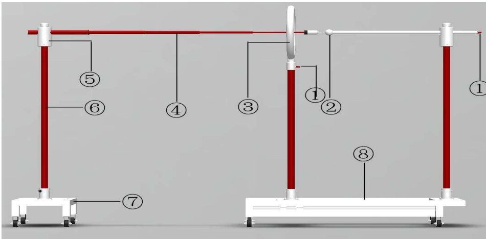
① 接线端子 ② 均压球 ③ 均压环 ④ 验电器 ⑤ 固定器 ⑥ 绝缘管 ⑦ 平车 ⑧ 带导轨平车
